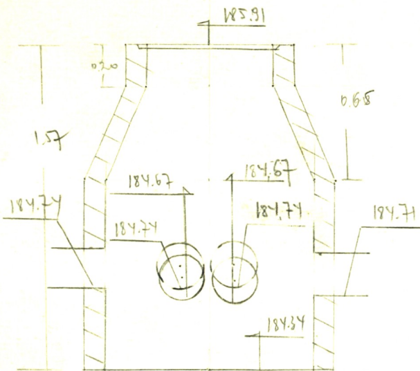
Šulinio brėžinys M 1:25
