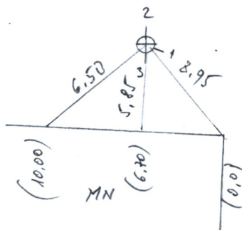
PRIRIŠIMO SCHEMA
