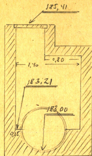
Чертеж колодца М 1:
