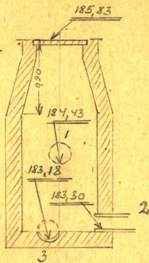
Чертеж колодца М 1:50
