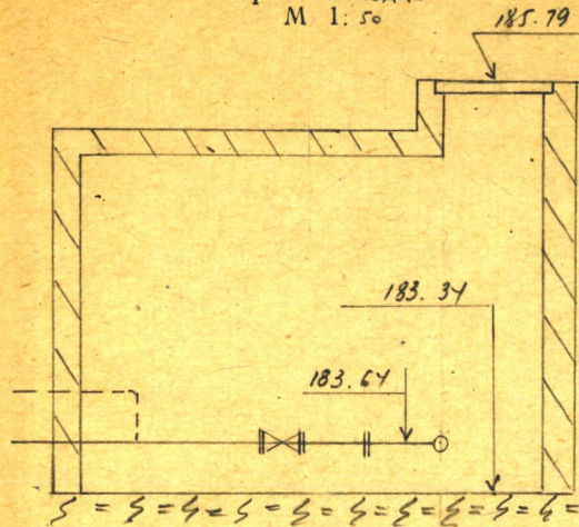
Чертеж колодца М 1:50
