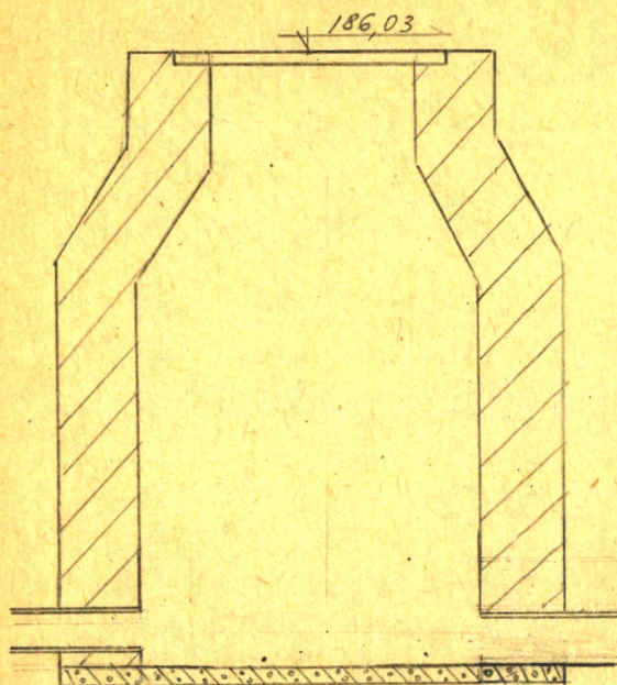
Чертеж колодца М 1:25
