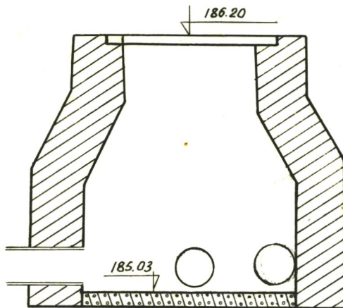
Чертеж колодца М 1:25
