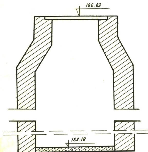
Чертеж колодца М 1:25
