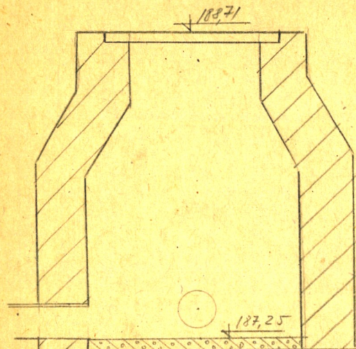
Чертеж колодца М 1:25
