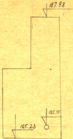
Чертеж колодца М 1:
