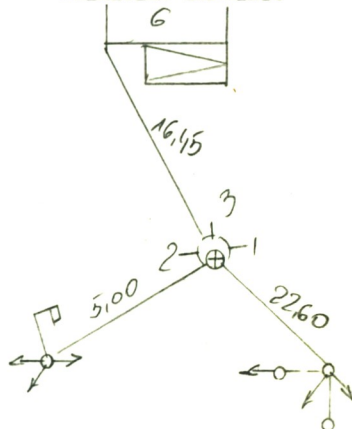
PRIRIŠIMO BRĖŽINYS
