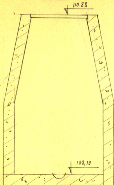
Чертеж колодца М 1:25
