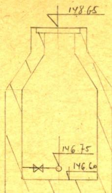
Чертеж колодца М 1:50
