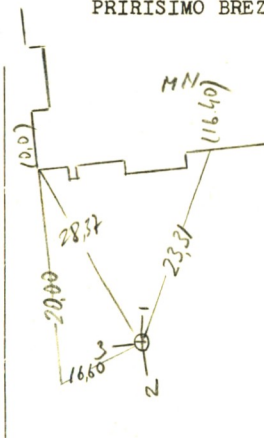
PRIRIŠIMO BRĖŽINYS
