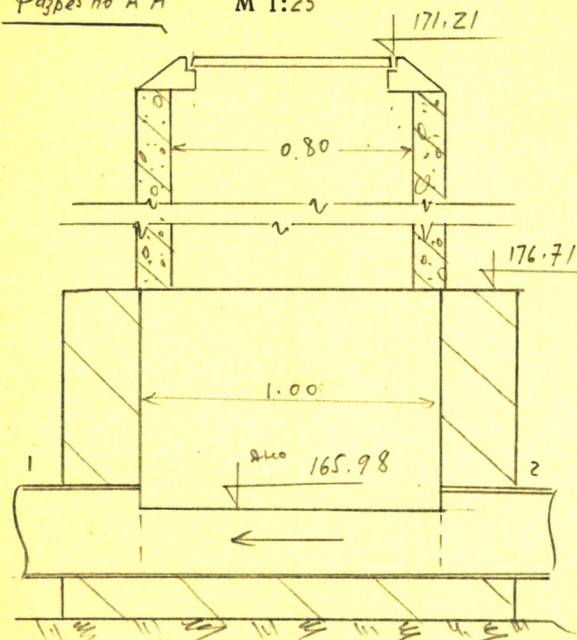
Чертеж колодца М 1:25 Разрез по А-А
