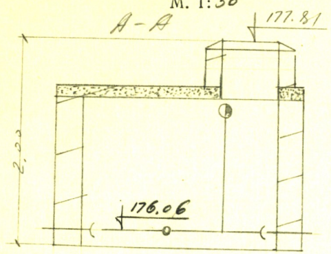
Чертеж колодца М. 1:50
