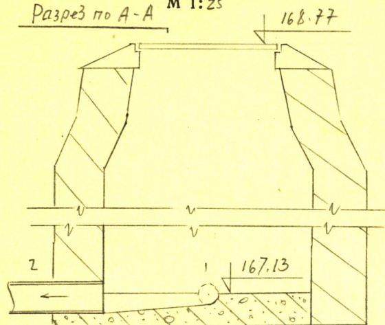
Чертеж колодца
