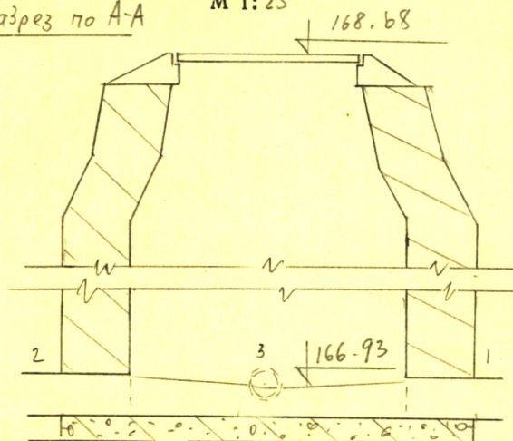
Чертеж колодца М 1:25
