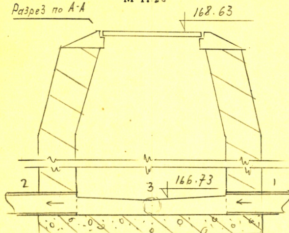
Чертеж колодца М 1:25
