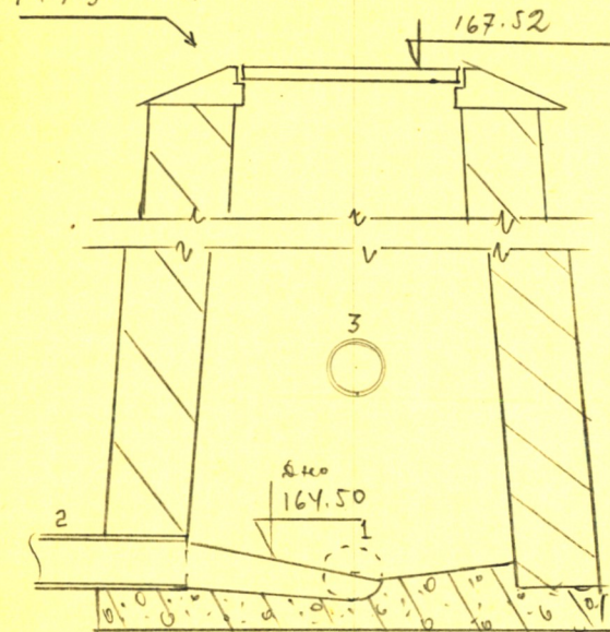
Чертеж колодца М 1:25 Разрез по А-А
