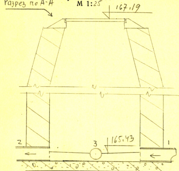
Чертеж колодца М 1:25 Разрез по А-А
