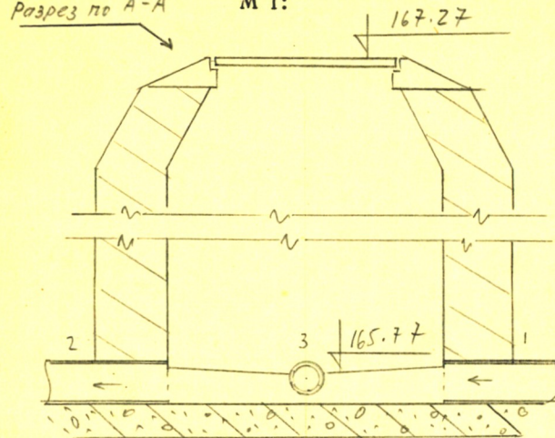
Чертеж колодца М 1: Разрез по А-А
