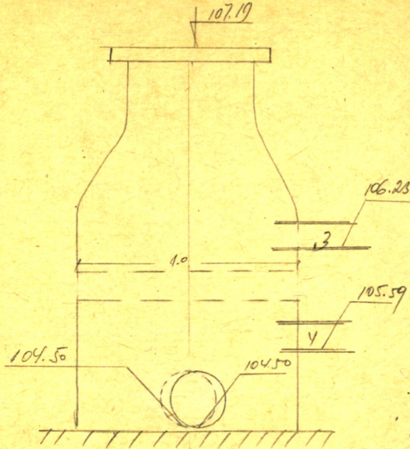
Чертеж колодца М 1:
