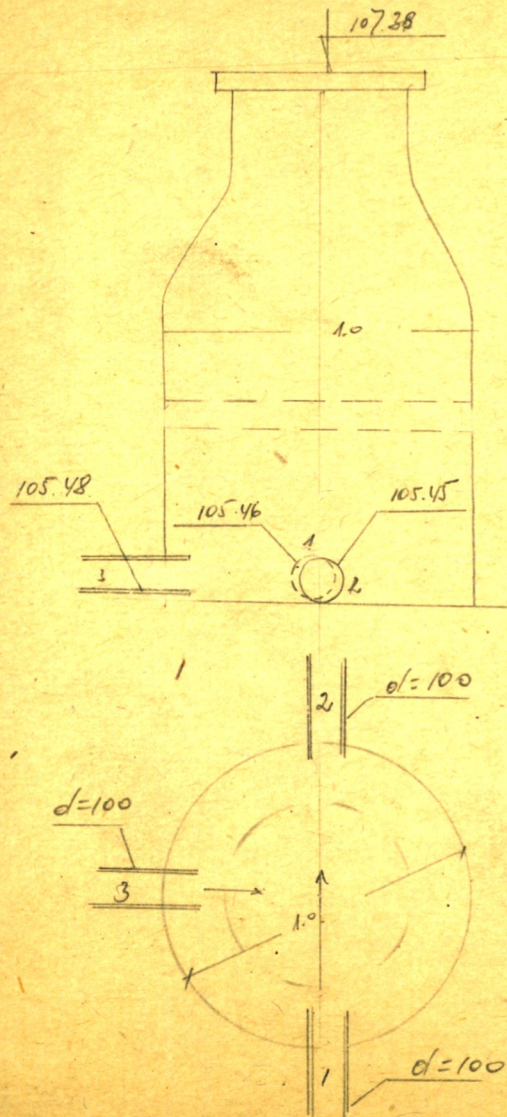
Чертеж колодца М 1:
