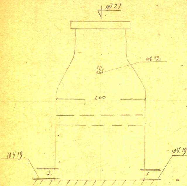
Чертеж колодца М 1:25
