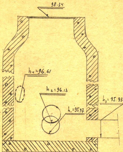
Чертеж колодца М 1:25
