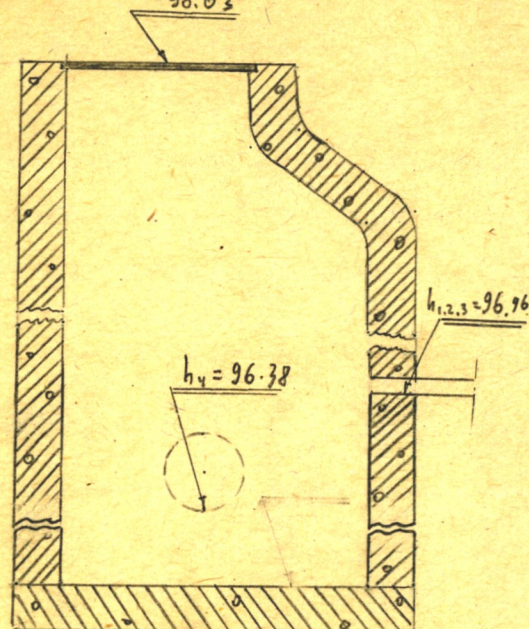
Чертеж колодца М 1:25 98.03
