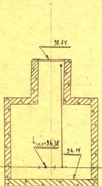
Чертеж колодца М 1:50
