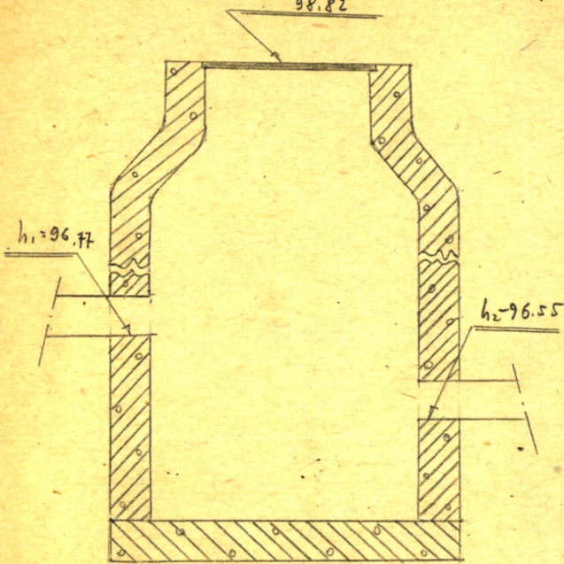
Чертеж колодца М 1:25 98.82
