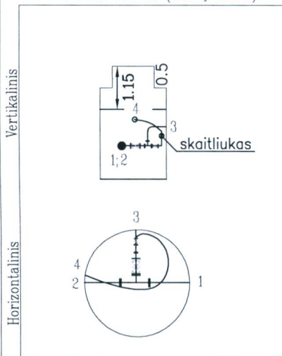
ŠULINIO PJŪVAI (Matmenys duoti m)
