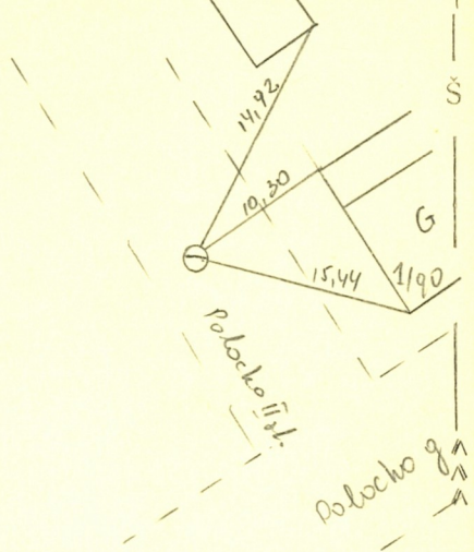
Pririšimo brėžinys:
