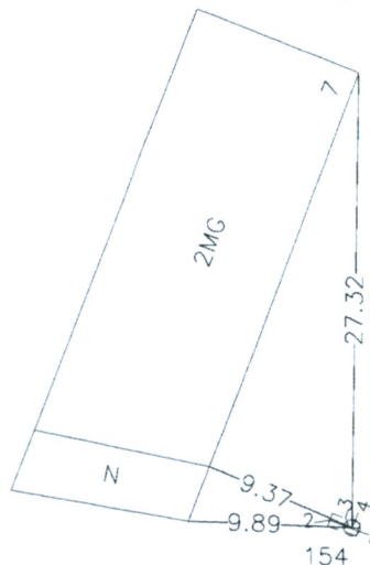
Pririšimo brėžinys
