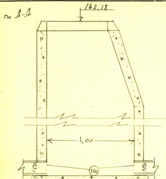
Чертеж колодца М 1
