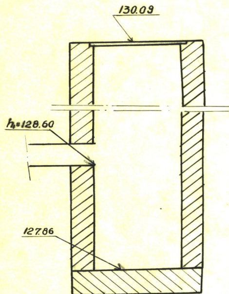
Чертеж колодца М1:25
