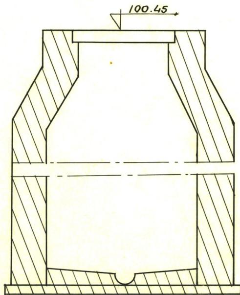
Чертеж колодца М 1:25
