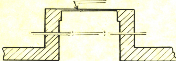
Чертеж колодца М1:25 129.69
