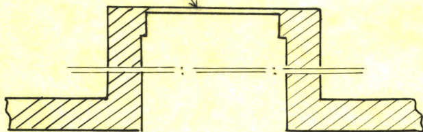
Чертеж колодца М 1:25
