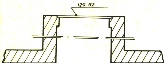
Чертеж колодца М1:25
