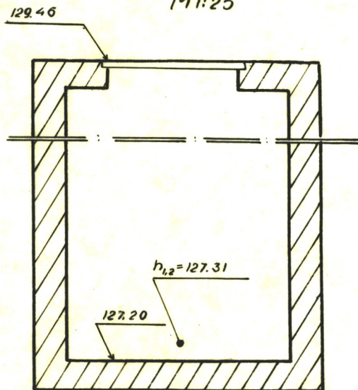
Чертеж колодца М 1:25
