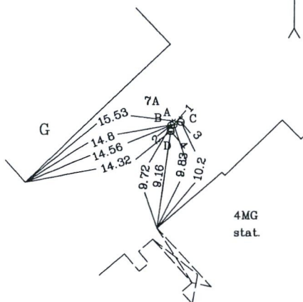
Pririšimo brėžinys
