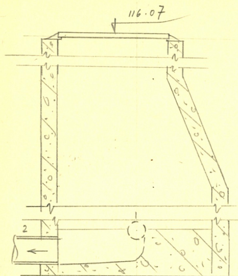
Чертеж колодца М 1:25
