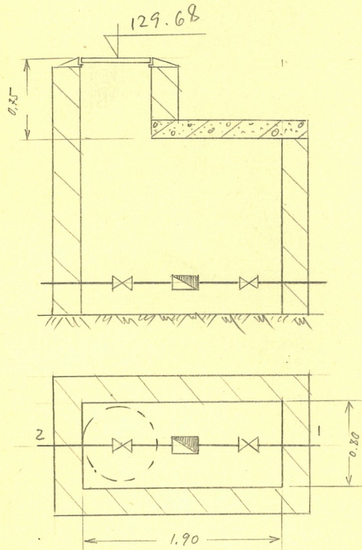
Чертеж колодца М. 1: 50
