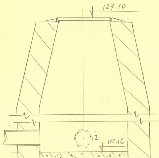
Чертеж колодца М 1: 25
