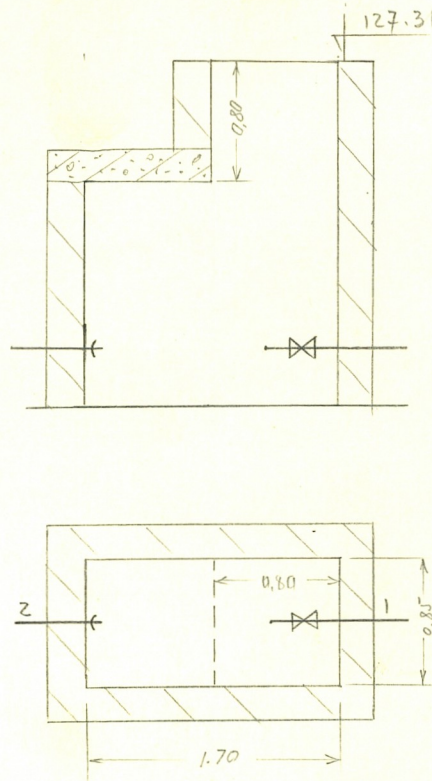
Чертеж колодца М. 1: 50
