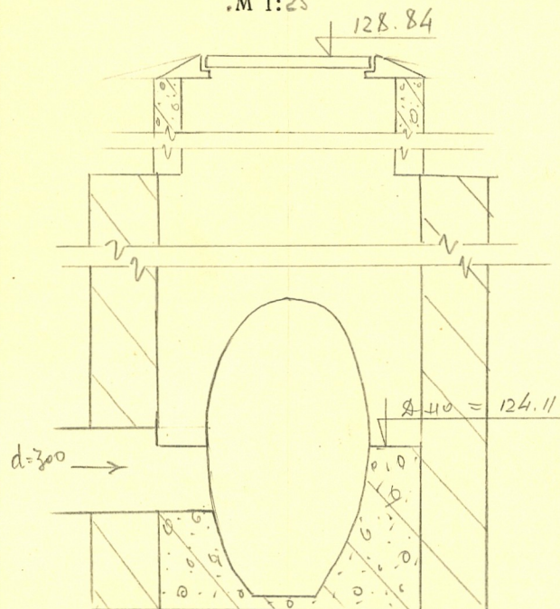
Чертеж колодца М 1:25
