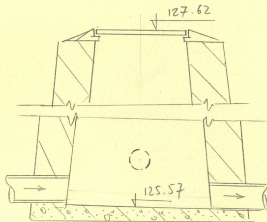
Чертеж колодца М 1:25
