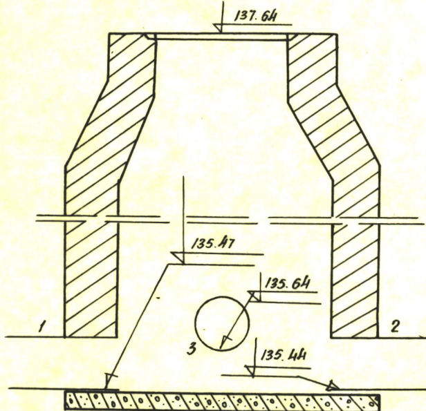
Чертеж колодца М 1:25
