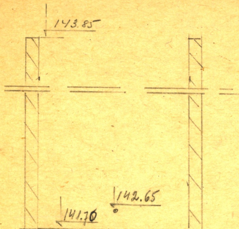
Чертеж колодца М 1:25
