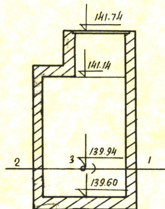
Чертеж колодезя М 1:50
