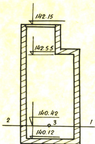
Чертеж колодца М 1:50
